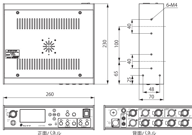
【ST#747BS 外観図】
